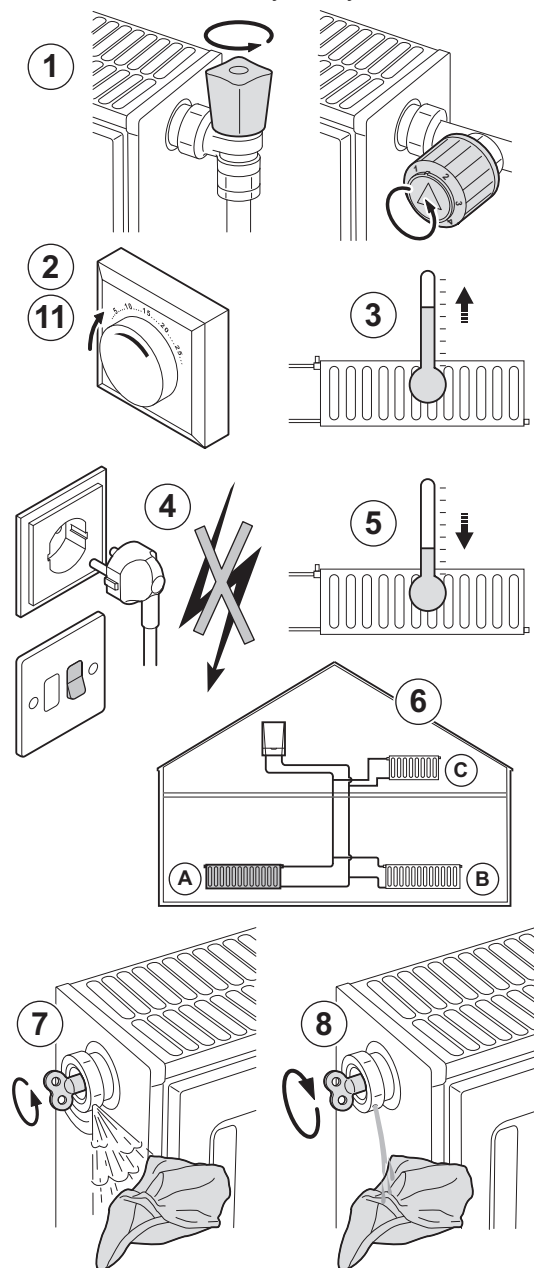
Рис.53 Удаление воздуха из установки
